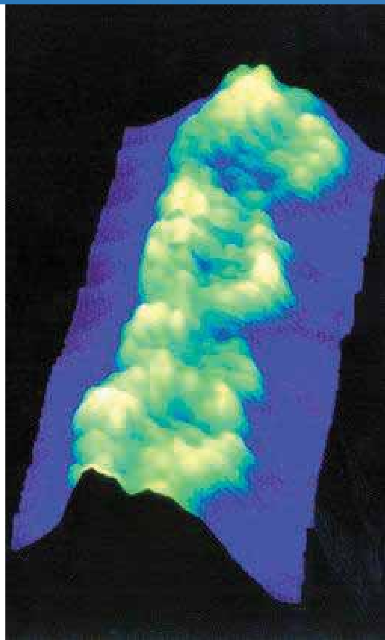
MICROFOTOGRAFÍA ELECTRÓNICA QUE MUESTRA PARTE DE UNA MOLÉCULA DE ADN. DE CIELO Y TIERRA (PHAIDON)
